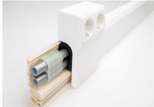
Slika 11. Instalcijski kanal Rauduo
